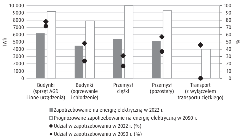
Rysunek 2. Obecne i prognozowane zapotrzebowanie na energię elektryczną w wybranych obszarach gospodarki światowej
